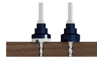
TerrassenFix® Bohrsenker BS 5 & BS 6
